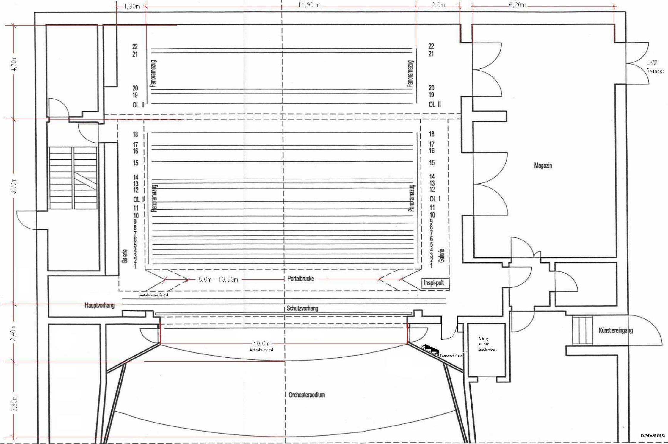
GRUNDRISS BÜHNE (PROSPEKTZÜGE) Theater in der Stadthalle Neumünster
